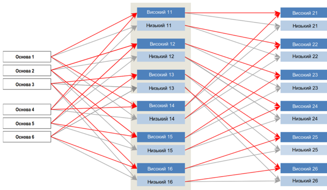
Рисунок I.A9.2. Багатоетапний дизайн адаптивного тестування із читання в PISA-2022: стандартний дизайн
