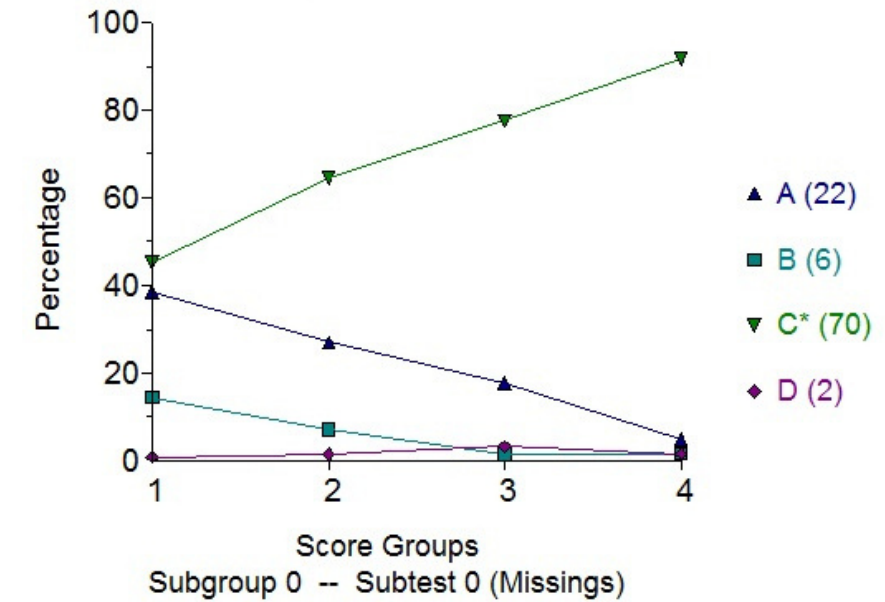
Item 32 z32 Rit = 0.4
