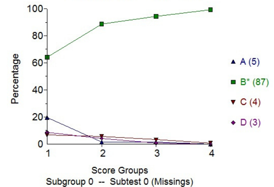
Item 79 z79 Rit = 0.43
